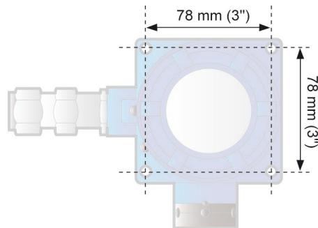
Figura 5: Sagoma di fissaggio della scatola
