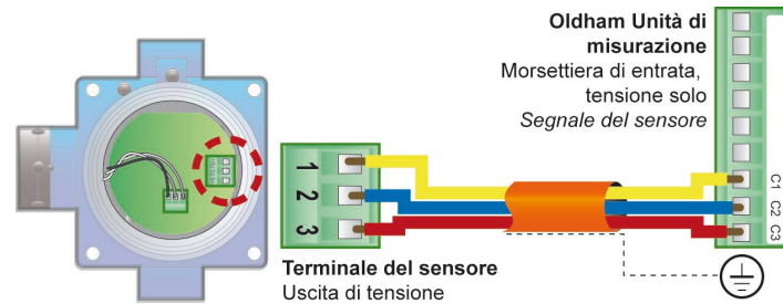
Figura 10: Connessioni per un rilevatore 3 cavi tipo OLC 100
