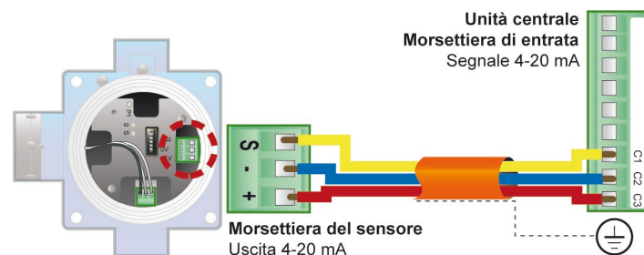
Figura 9: Connessioni per un rilevatore 4-20 mA 3 cavi
