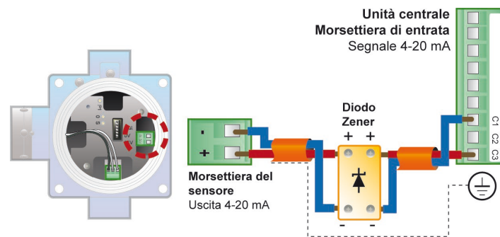
Figura 8 : Connessioni per un rilevatore di sicurezza intrinseco 4-20 mA 2 cavi con barriera a diodi Zener
