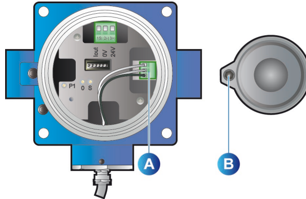
Figura 16: OLCT 100 HT – elementi specifici relativi alla sostituzione della cella alta temperatura.
