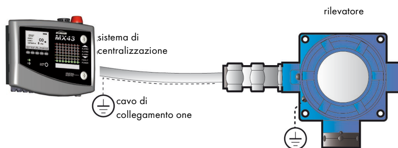
Figura 6: Il cavo di collegamento che collega il rilevatore del sistema di centralizzazione deve essere scelto con attenzione
