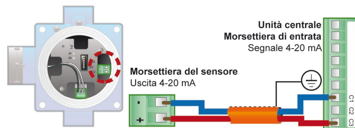
Figura 7: Connessioni per un rilevatore 4-20 mA 2 cavi
